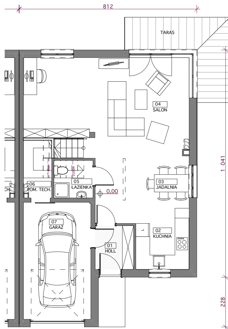
RZUT PARTERU
